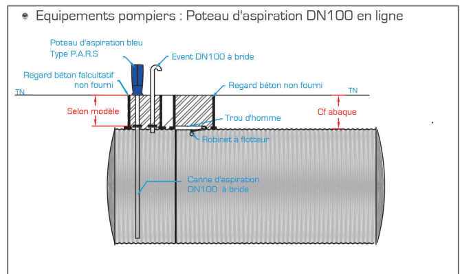
Réserve galvanisée enterrée Vue de profil
