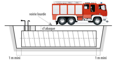
Réserve galvanisée enterrée Vue de profil
